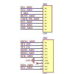
Arduino-LR2012 Headers
