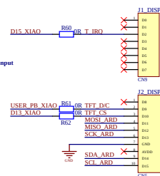
DM-TFT28-116 Display Header (optional)
