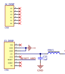
DM-TFT28-116 Display Header (optional)
