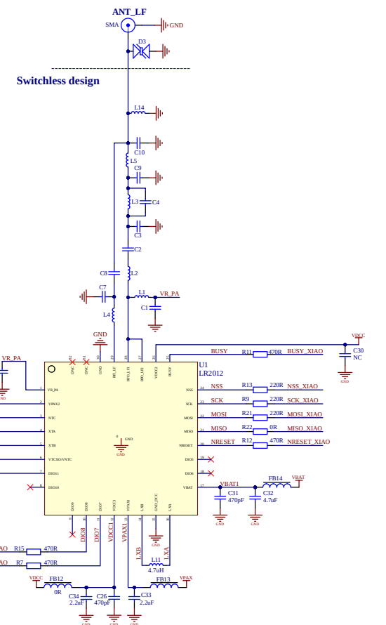
ANT_LF SubGHz - 490MHz
